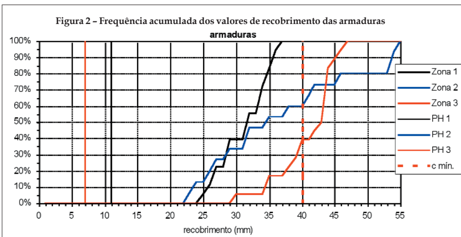
Representação gráfica da frequência acumulada do valores de recobrimento das armaduras, medidos com o pacómetro, da profundidade de carbonatação do betão e recobrimento mínimo regulamentar, em várias zonas de ensaio.
